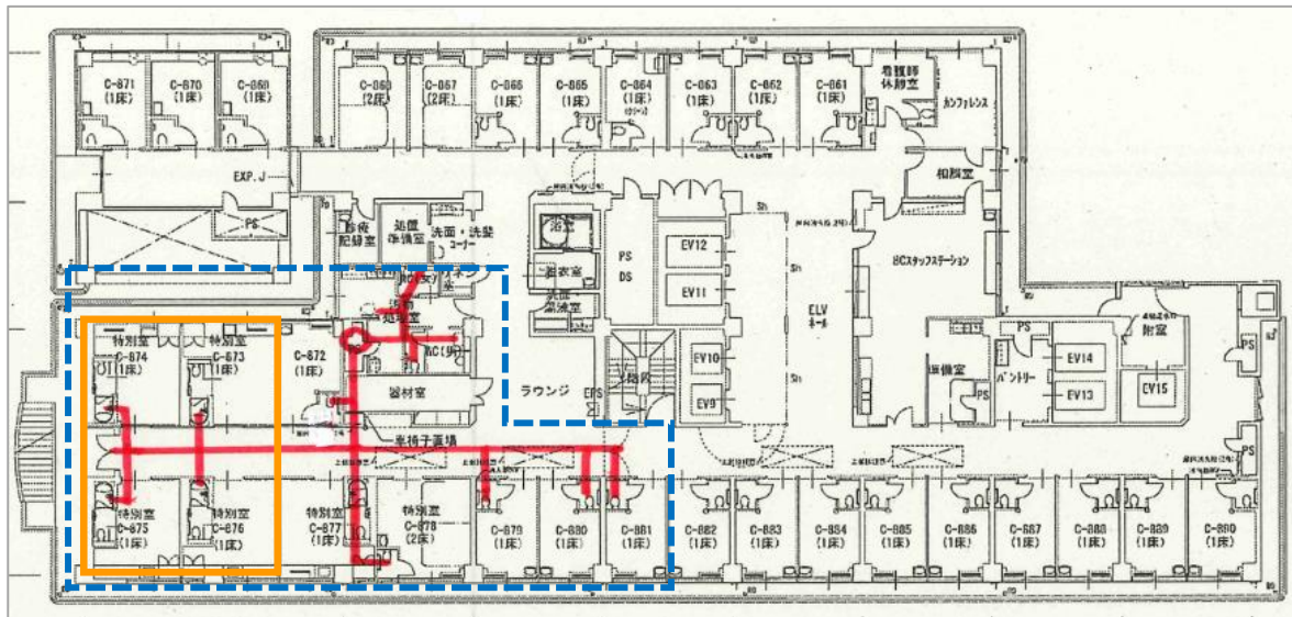
西館 8 階病棟図面
