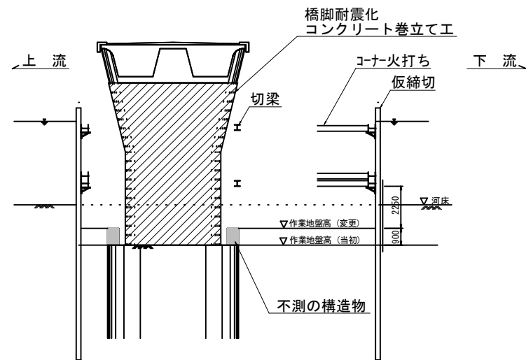
橋脚断面図
