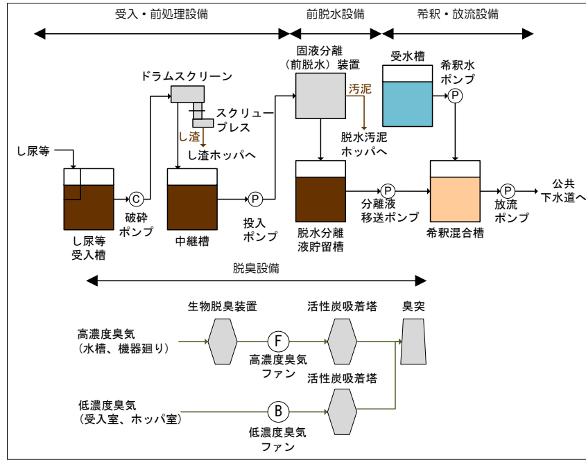
「前脱水+汚泥助燃剤化+希釈放流方式」処理フロー図
