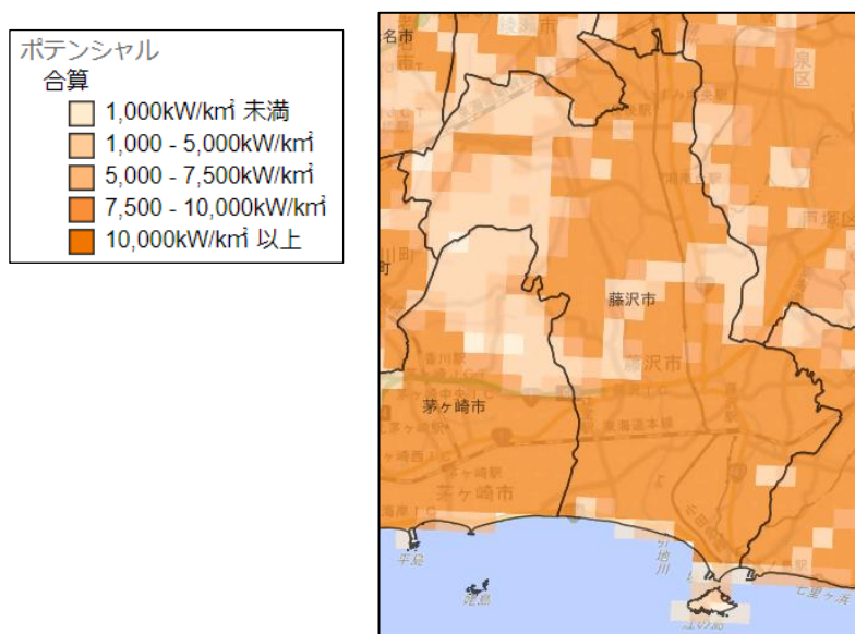
図 2-5 太陽光発電設備のポテンシャルの分布 (建物系)
