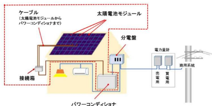
図2-3 太陽光発電の構成
