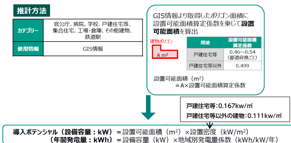
図 2-4 REPOS による太陽光発電設備の導入ポテンシャルの算定方法
